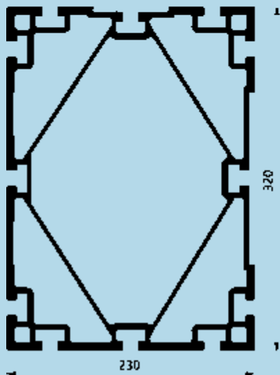
NTS 32x23 I die No. 41741 G=34,65 kg/m
